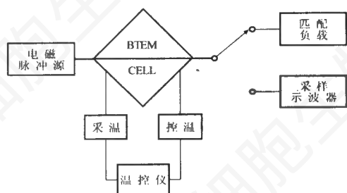
图1 实验系统图
