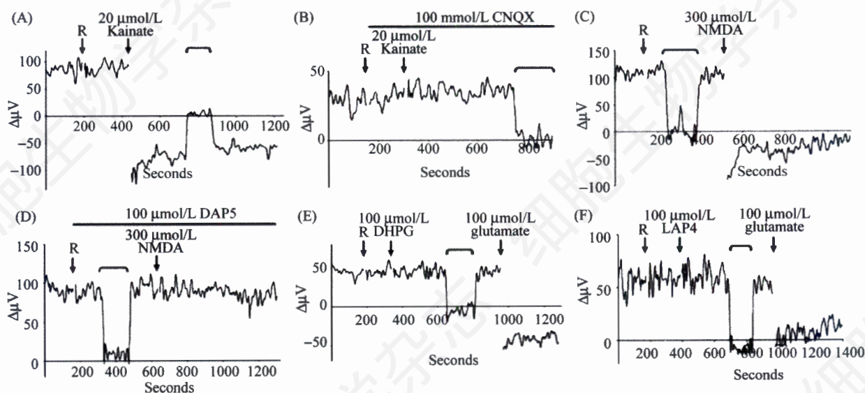
图 1 通过测量单个鲶鱼水平细胞的胞外 H^+ 流表征谷氨酸受体兴奋剂的作用 [3]
